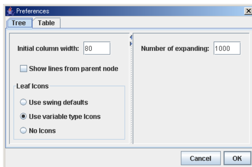
図 21: Preference/TreeView タブ
